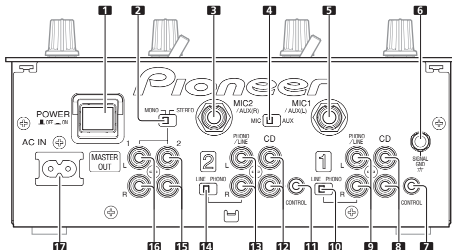
Rückwand
