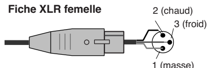
Fiche XLR femelle
