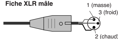
Fiche XLR mâle
