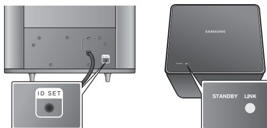
<Vue arrière du caisson de basses> <Vue avant du caisson de basses>
