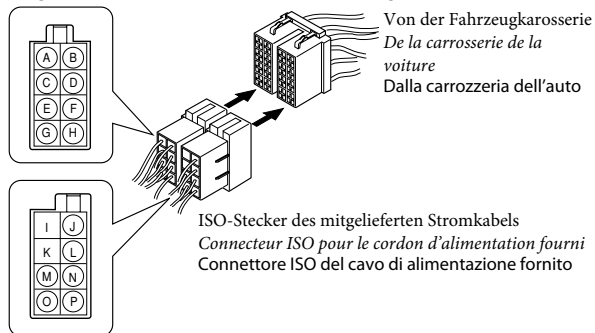
Von der Kabelseite aus gesehen Vue à partir du côté des fils Vista dal lato dei cavi
