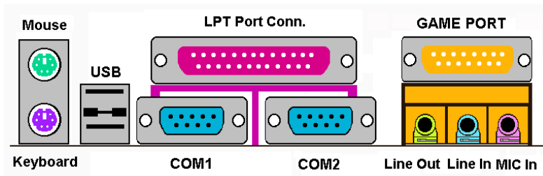
Figure 2-13. Disposition des connecteurs arrière de la VH6
