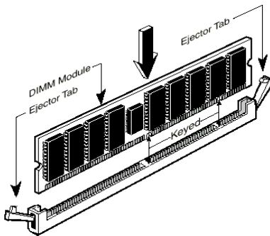
Figure 2-6. Installation d'une mémoire
