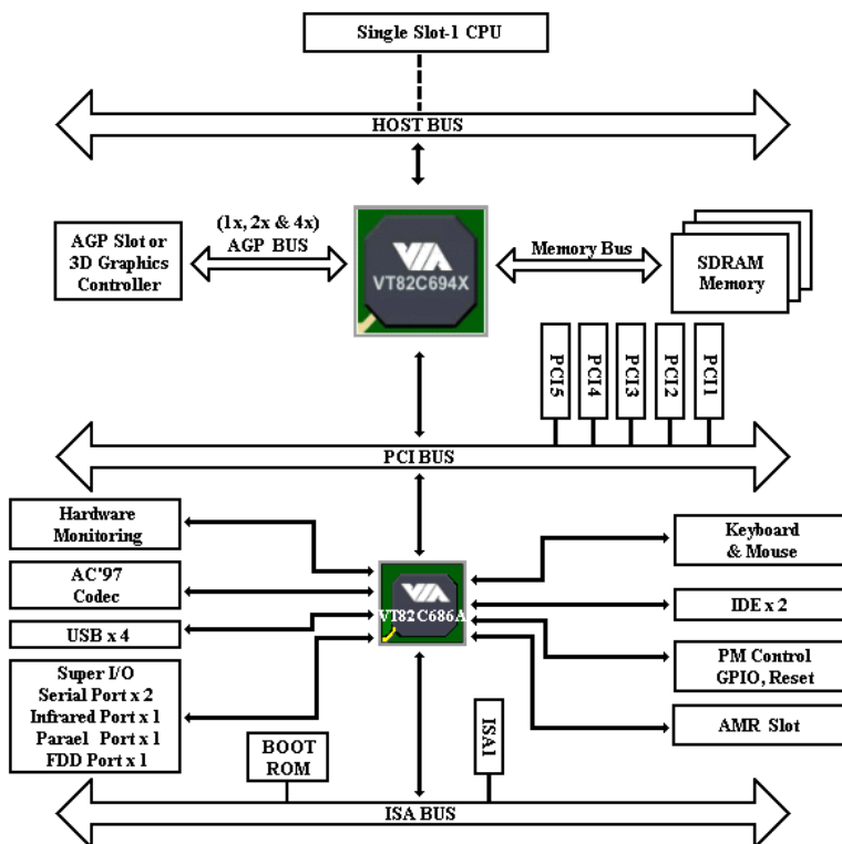
Figure 1-3. diagramme Système du chipset VIA Apollo Pro 133A
