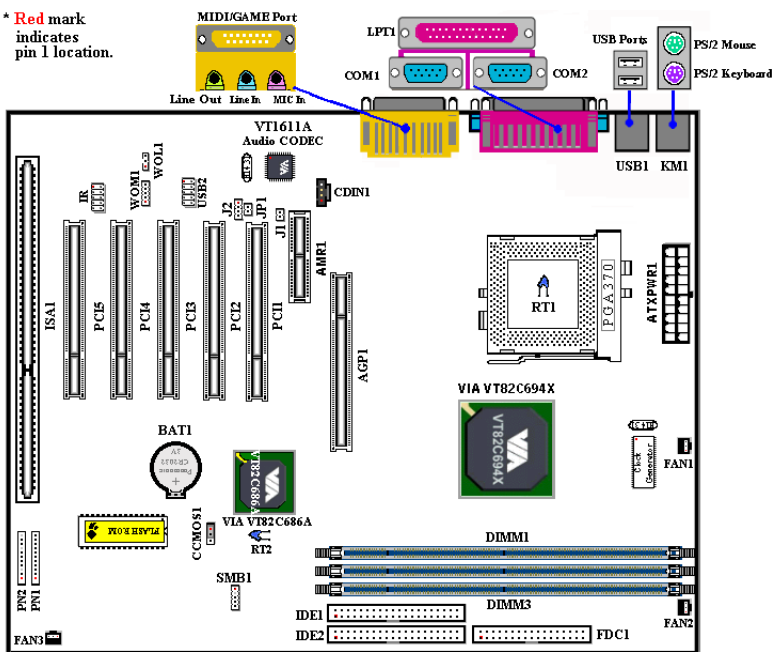
Figure 1-2. Disposition des composants de la carte mère
