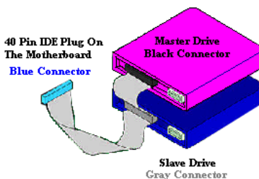
Figure 2-12. Comment connectez la nappe Ultra ATA/66 sur votre carte mère
