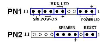
Figure 2-9. définitions des pins du PN1 et PN2
