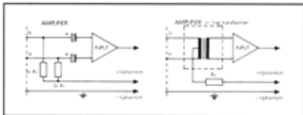
Abb. 5: Phantomspaltung bei asymmetrischen Eingängen
