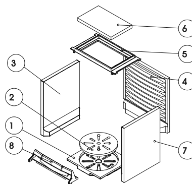
Numerazione dei refrattari = istruzioni di montaggio
