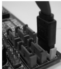
Collegare il cavo dati SATA al connettore SATAII arancione (SATAII_6 (PORT3.1))
