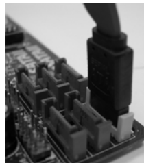
SATA データケーブル をオレンジ SATAII コネク タ (SATAII_6 (PORT3.1)) に接続します
