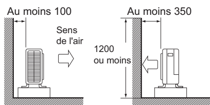
Vue latérale
