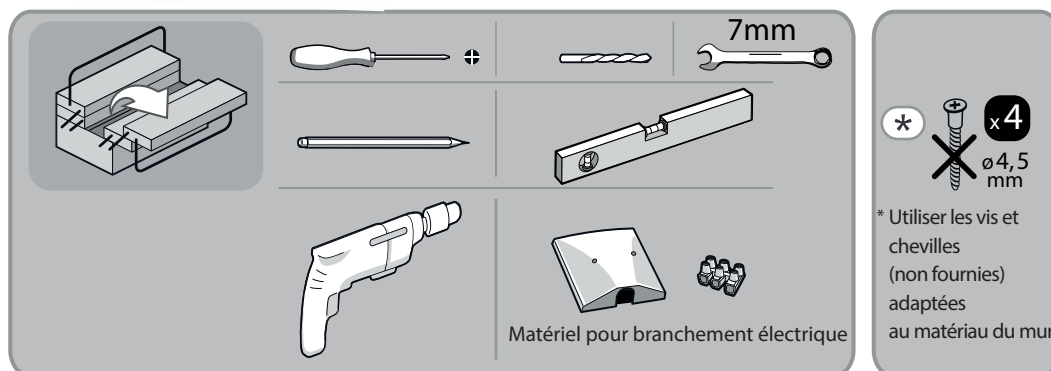
Matériel nécessaire au montage du radiateur.
