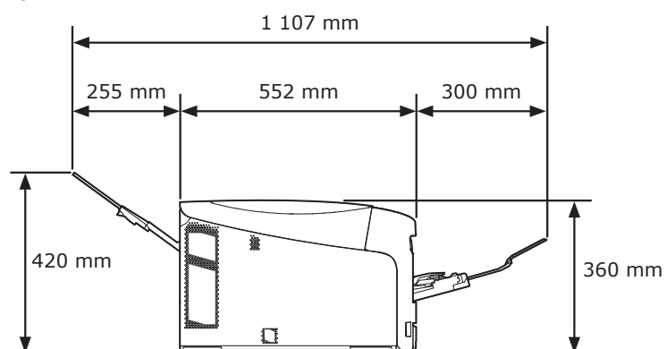
VUE LATÉRALE
