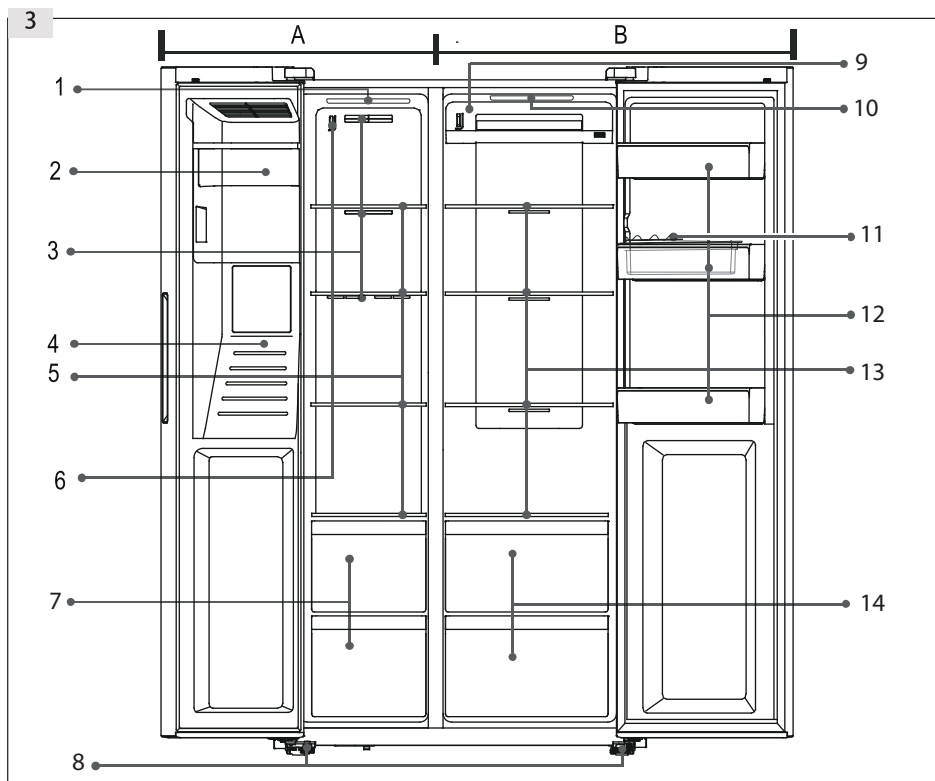
Schéma de l'appareil (Fig. 3)
