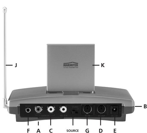
Image 3 EMETTEUR A/V
