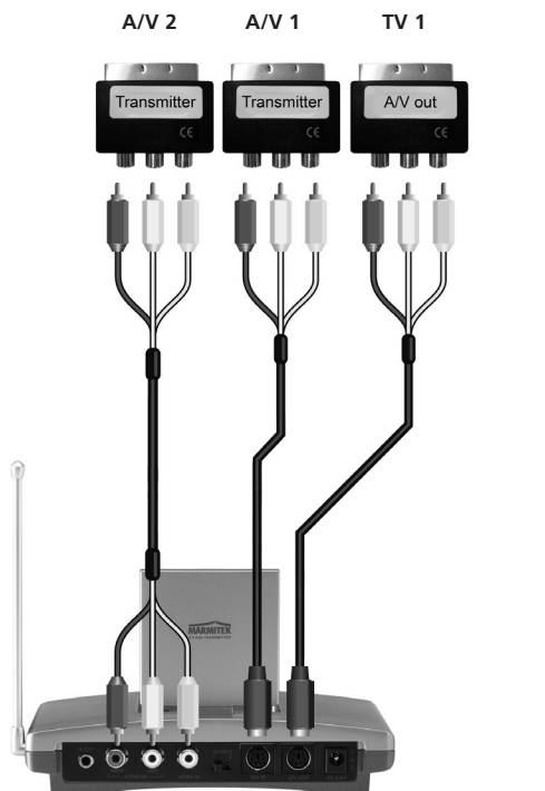
Abbildung 1 A/V SENDER
