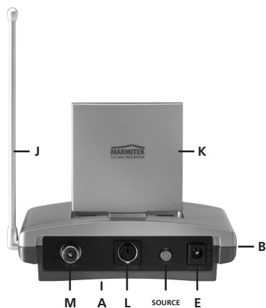
Abbildung 4 A/V EMPFÄNGER
