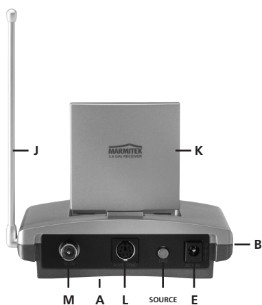
Afbeelding 4 A/V ONTVANGER
