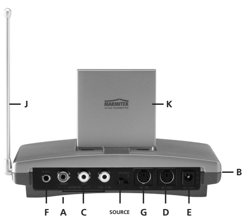
Afbeelding 3 A/V ZENDER
