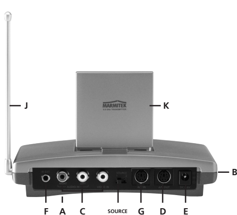
Abbildung 3 A/V SENDER
