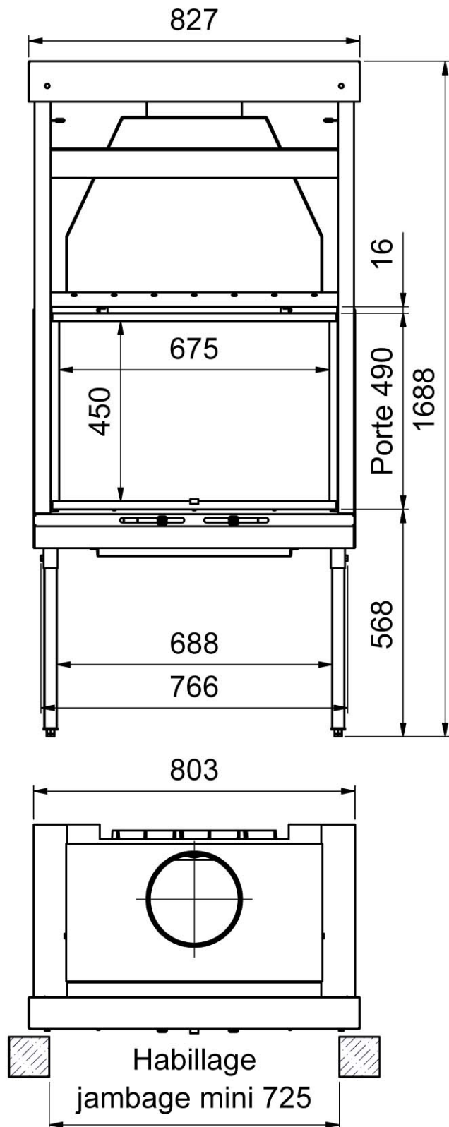
Foyer STELLA2 PORTE ESCAMOTABLE Dimensions hors tout utiles L 830 x H 1690 x P 510 mm
