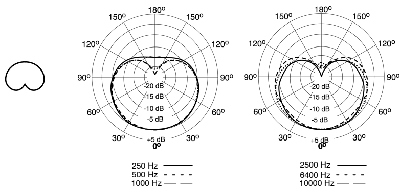
FIGURE 4. COURBES DE DIRECTIVITÉ TYPIQUES
