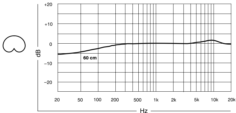
FIGURE 3. RÉPONSE EN FRÉQUENCE TYPIQUE
