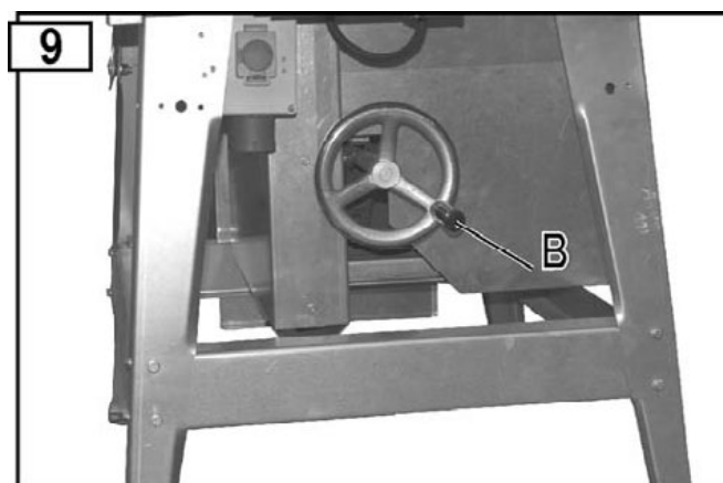
Réglage de la hauteur de coupe type BTH La hauteur de coupe se règle en tournant le volant (B). Le réglage de la hauteur de coupe souhaitée s'effectue en continu.
