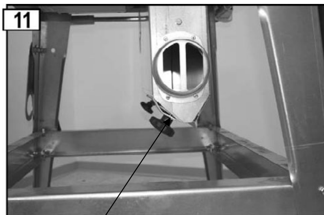
Spanauswurfschlitzen offen (Betrieb ohne Späneabsaugvorrichtung)
