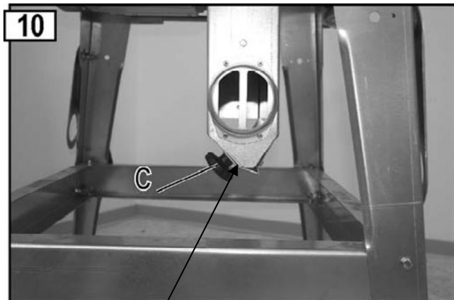
Spanauswurfschlitzen geschlossen (Betrieb mit Späneabsaugvorrichtung)
