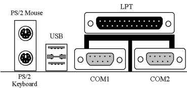
Figure 2-8. Connecteurs d’entrées/sorties de votre BX6.
