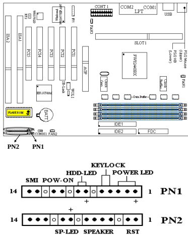
Figure 2-7. Définitions des pins du PN1 et PN2
