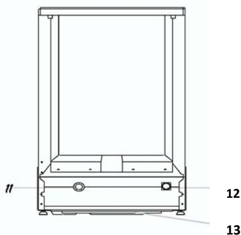
Vue Arrière
