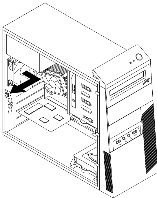
Figure 56. Retrait du bloc de ventilation arrière
