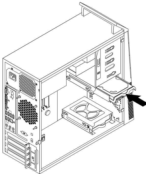
Figure 50. Installation de l'unité de disque dur principale
