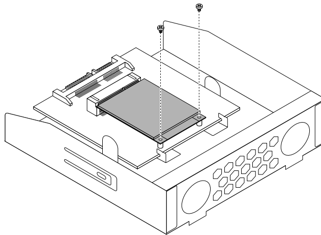
Figure 46. Installation des vis de fixation de l'unité SSD mSATA
