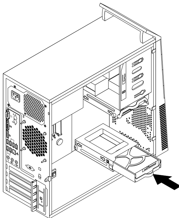
Figure 53. Installation de l'unité de disque dur secondaire
