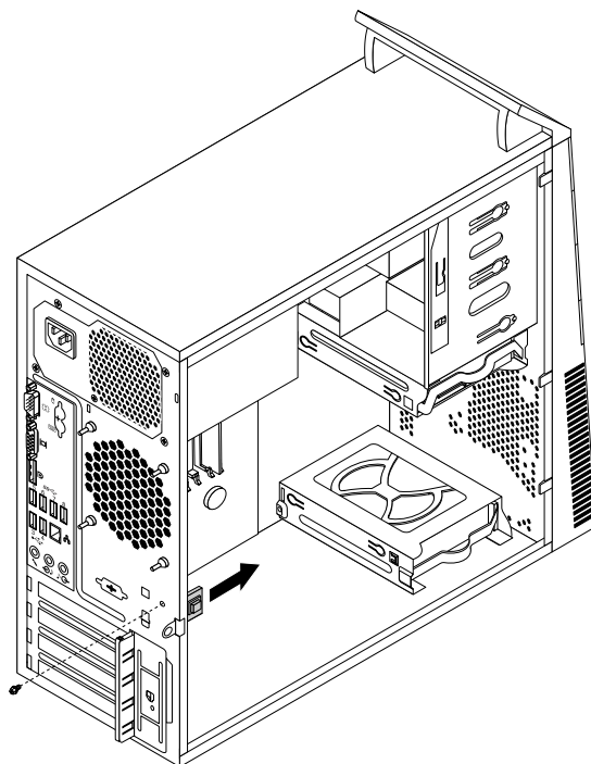
Figure 63. Retrait de l'interrupteur de détection de présence du carter
