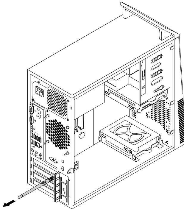
Figure 75. Retrait de l'antenne WiFi arrière
