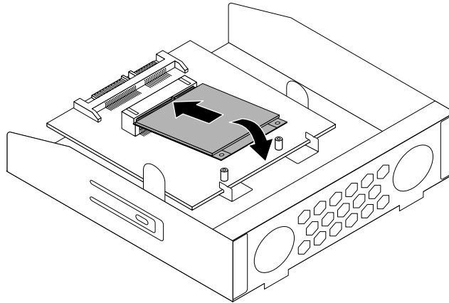
Figure 39. Installation de l'unité SSD mSATA dans le convertisseur de stockage
