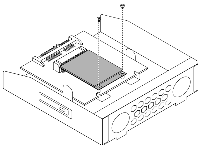
Figure 43. Retrait des vis de fixation de l'unité SSD mSATA
