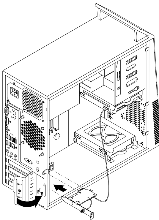
Figure 73. Installation de la carte d'interface WiFi
