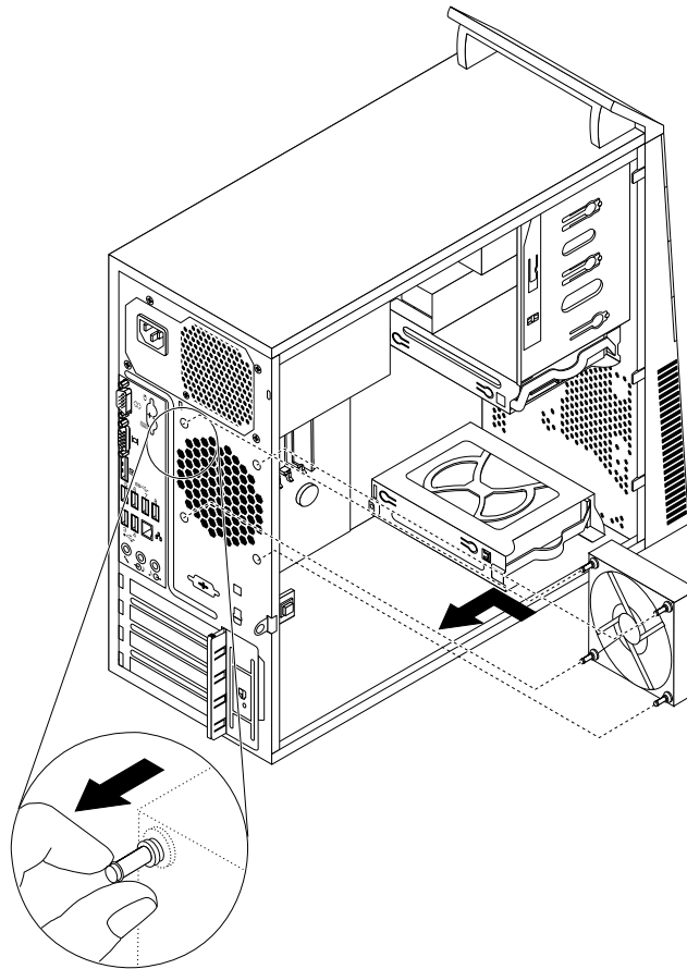
Figure 57. Installation du bloc de ventilation arrière
