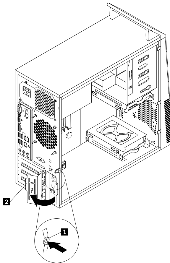
Figure 13. Ouverture du loquet de la carte PCI
