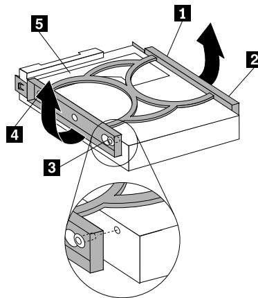
Figure 49. Installation de l'unité de disque dur dans le système de retenue
