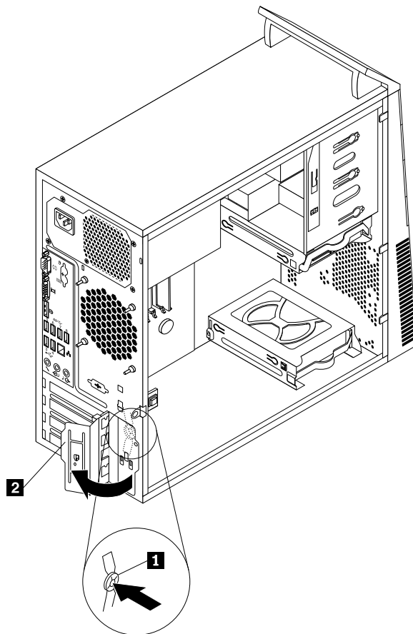
Figure 66. Ouverture du loquet de la carte PCI
