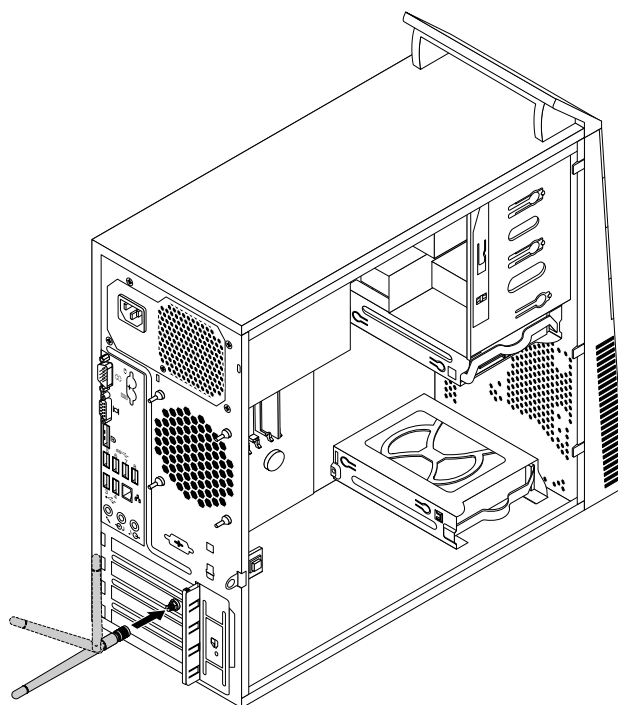
Figure 74. Installation de l'antenne WiFi arrière
