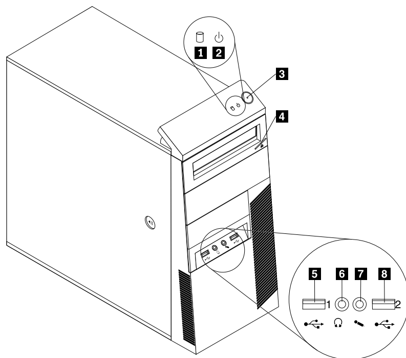
Figure 1. Emplacement des connecteurs, des boutons de commande et des voyants à l'avant
