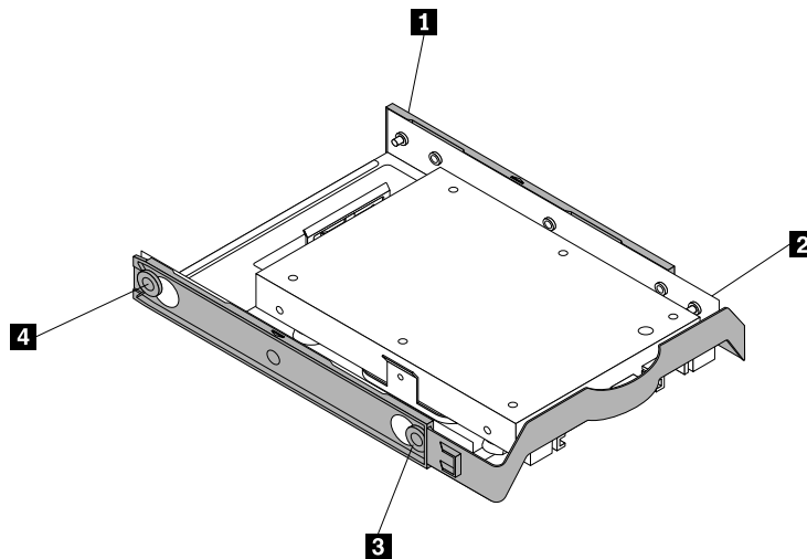
Figure 38. Installation de l'unité SSD avec le convertisseur de stockage dans le support de l'unité de disque dur
