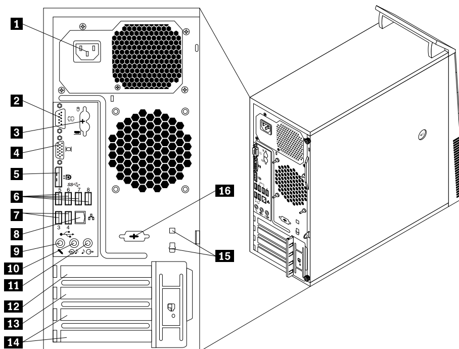
Figure 2. Emplacement des connecteurs à l'arrière
