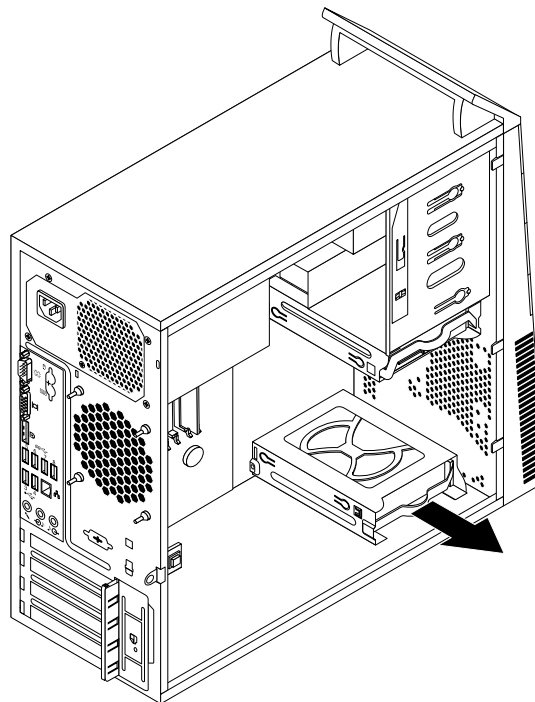
Figure 51. Retrait de l'unité de disque dur secondaire
