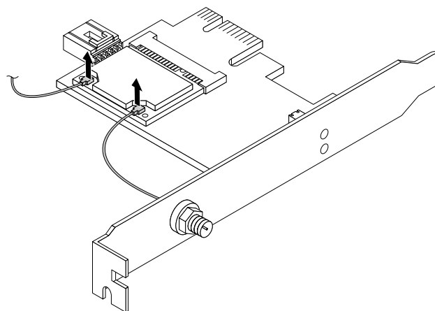
Figure 68. Retrait des câbles d'antennes WiFi
