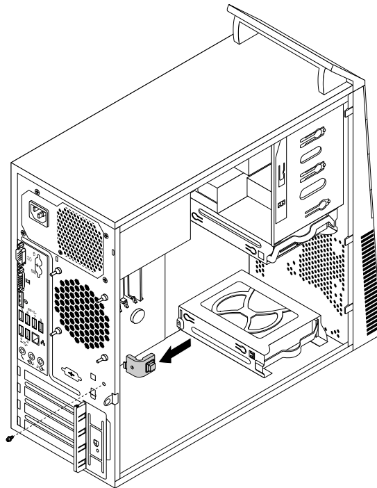
Figure 64. Installation du nouvel interrupteur de détection de présence
