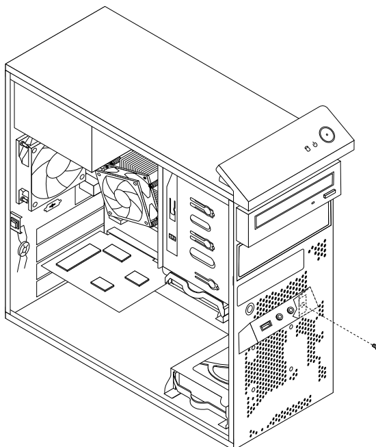
Figure 58. Retrait de la vis qui permet de fixer le bloc audio/USB avant au boîtier
