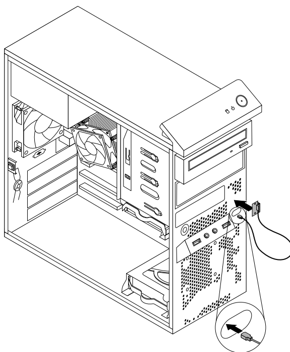
Figure 77. Installation de l'antenne WiFi avant
