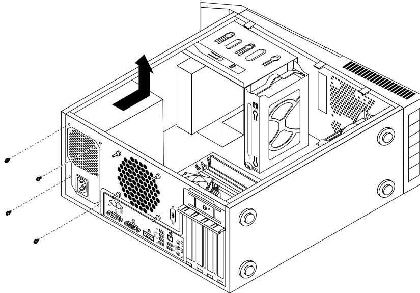
Figure 32. Retrait des vis de fixation du bloc d'alimentation électrique
