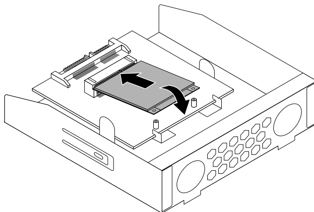
Figure 45. Installation de l'unité SSD mSATA dans le convertisseur de stockage
