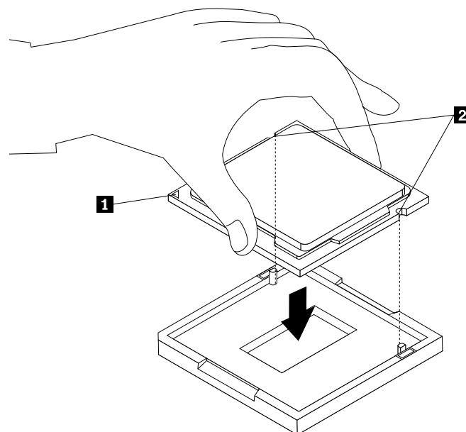
Figure 36. Installation du microprocesseur
