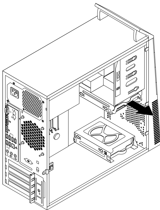
Figure 48. Retrait de l'unité de disque dur principale
