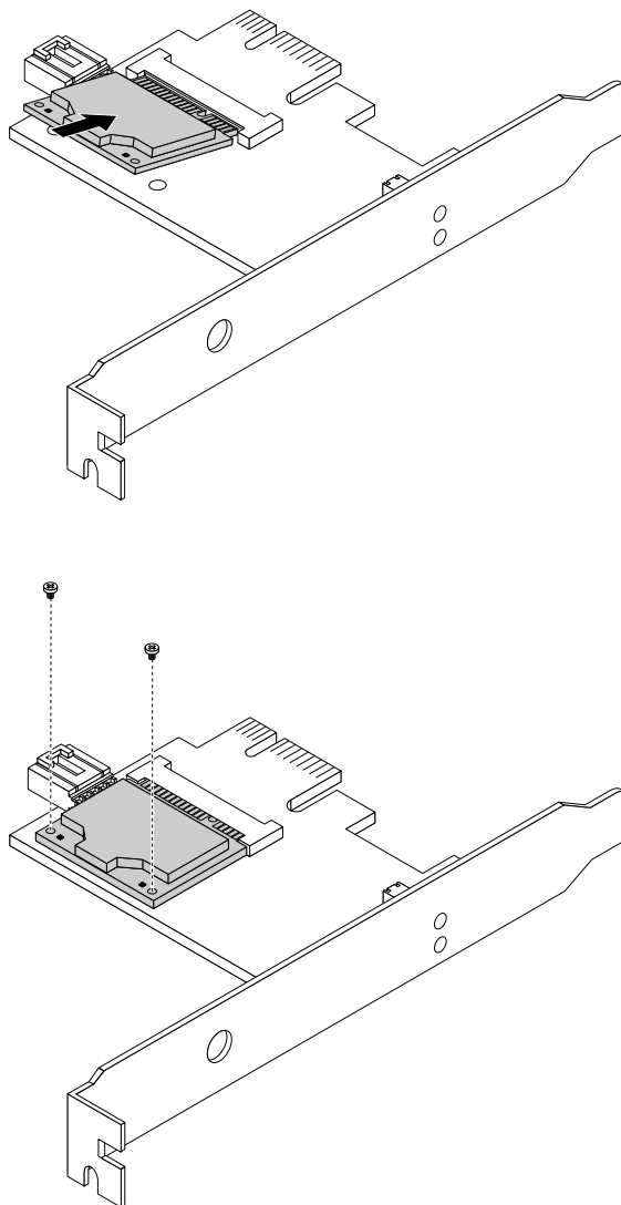
Figure 71. Installation du module de carte WiFi
