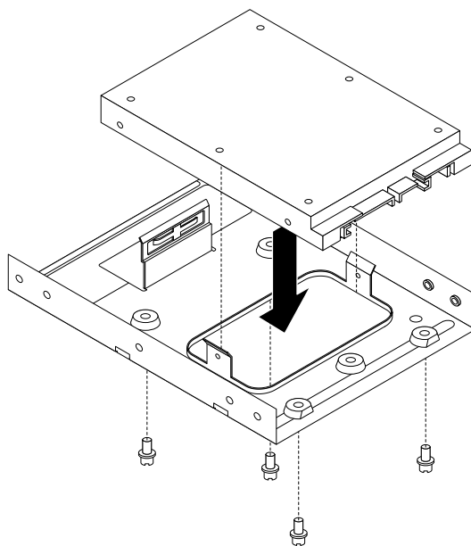
Figure 37. Installation de l'unité SSD dans le convertisseur de stockage
