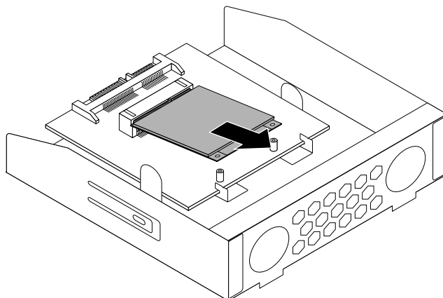
Figure 44. Retrait de l'unité SSD mSATA
