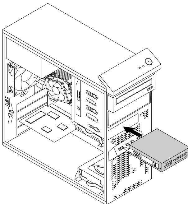
Figure 25. Installation du lecteur de cartes
