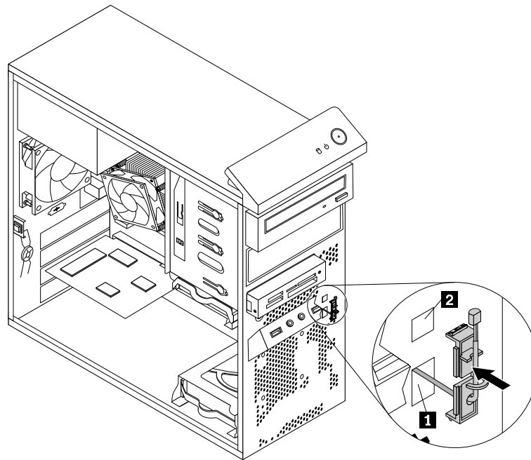
Figure 62. Installation du nouveau capteur thermique
