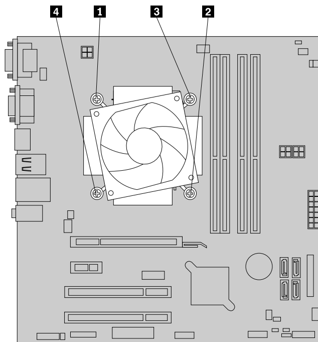
Figure 33. Retrait du dissipateur thermique et du bloc de ventilation
