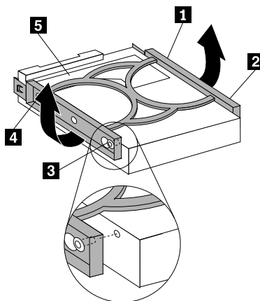
Figure 52. Installation de l'unité de disque dur dans le système de retenue
