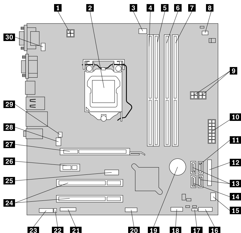
Figure 5. Emplacements des composants sur la carte mère
