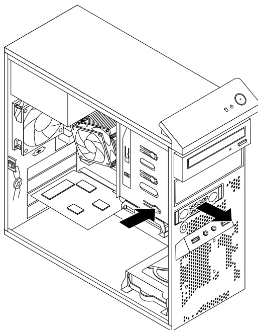
Figure 42. Retrait du convertisseur de stockage de l'unité SSD mSATA
