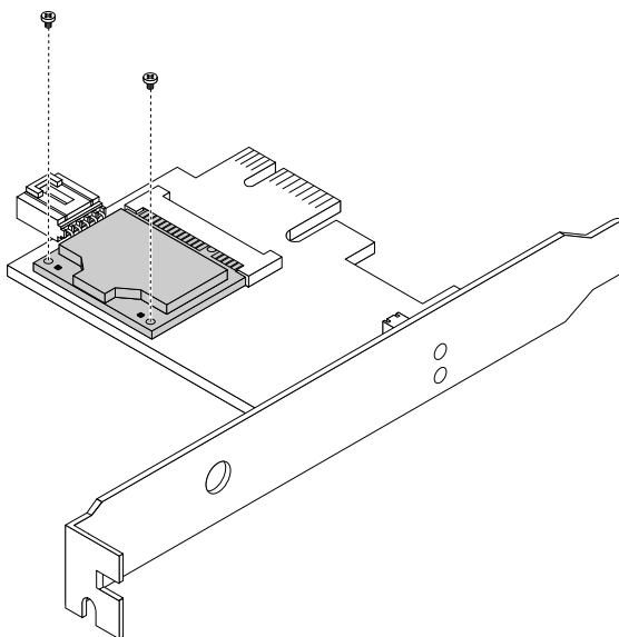
Figure 69. Retrait des vis de fixation du module de carte WiFi
