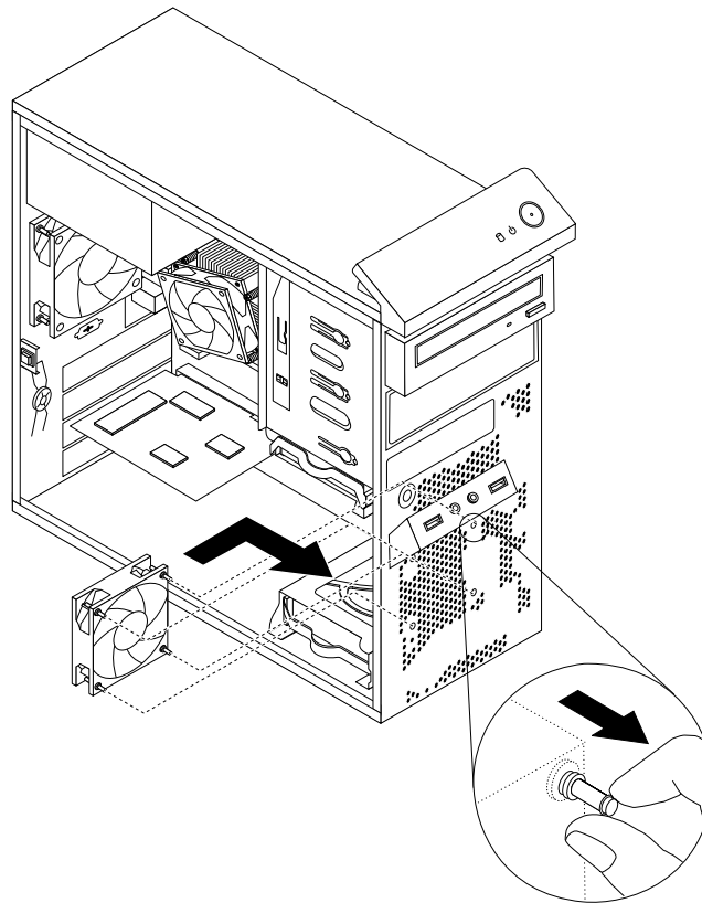
Figure 55. Installation du bloc de ventilation avant
