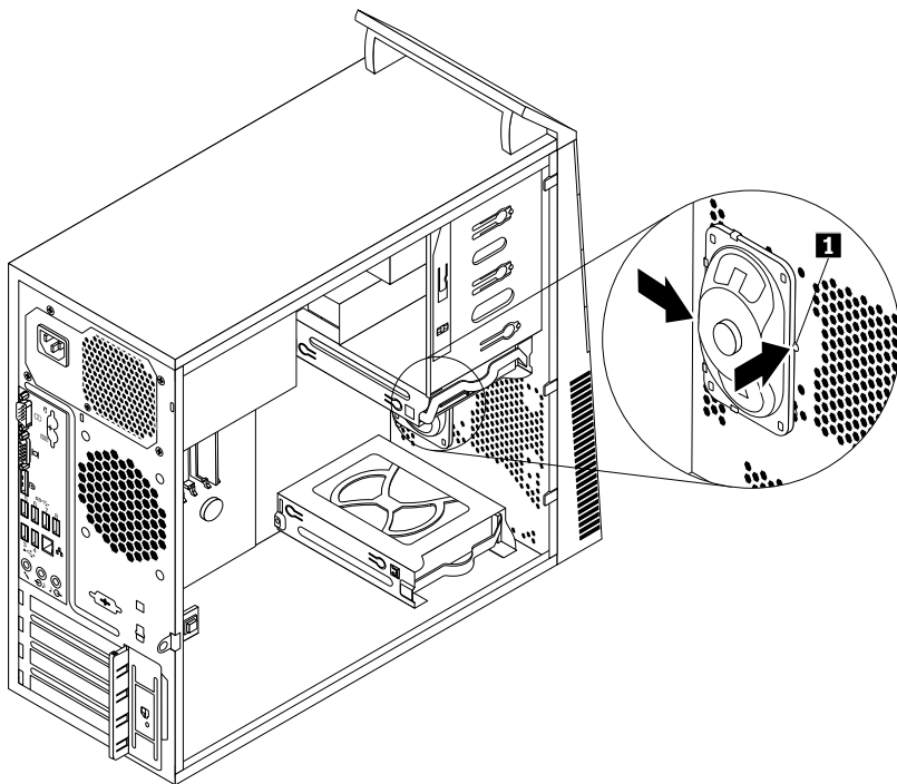
Figure 59. Retrait de l'ancien haut-parleur interne
