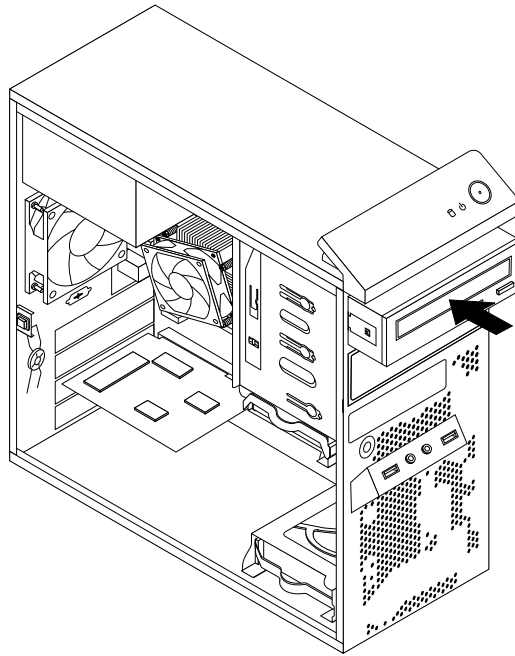
Figure 21. Installation de l'unité de disque optique
