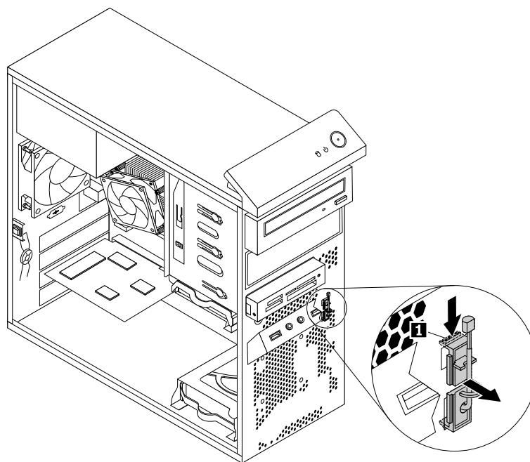
Figure 61. Retrait du capteur thermique
