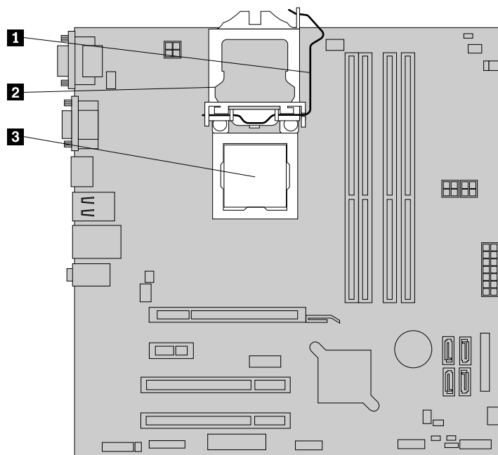
Figure 34. Accès au microprocesseur
