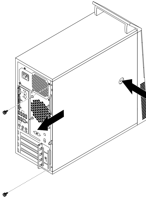
Figure 11. Retrait du carter de l'ordinateur
