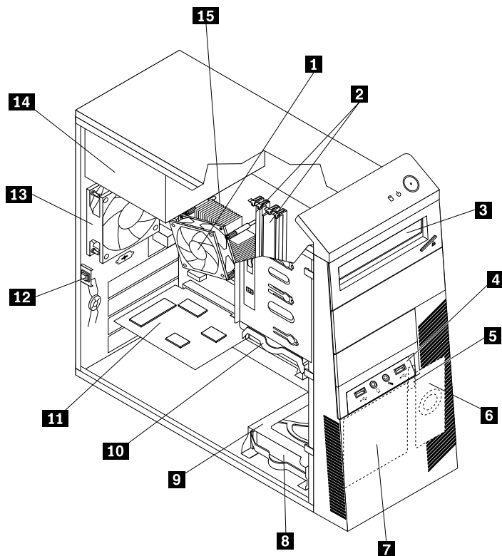
Figure 3. Emplacement des composants
