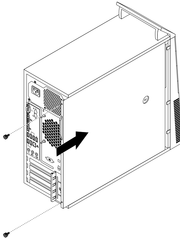
Figure 80. Remise en place du carter de l'ordinateur
