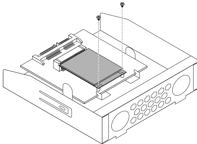
Figure 40. Installation des vis de fixation de l'unité SSD mSATA
