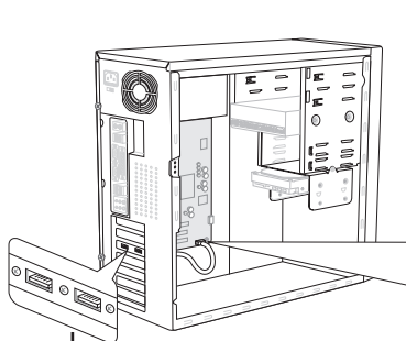
Кронштейн USB 3.0 (дополнительно)
