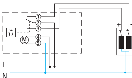
RAM 7.. commande la vanne mélangeuse motorisée
