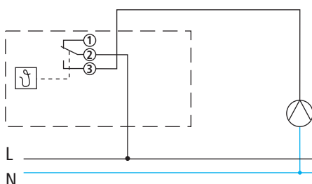
RAM 784 pilote la pompe de circulation ou le brûleur à gaz/à mazout
