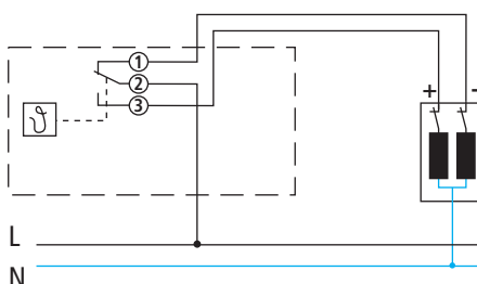
RAM 784 commande la vanne mélangeuse motorisée
