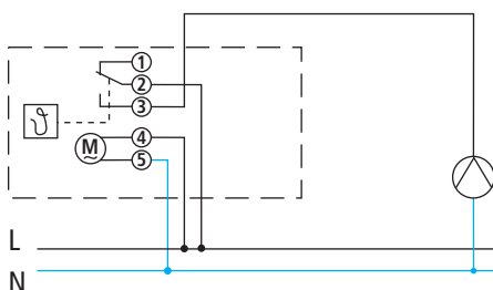
RAM 7.. pilote la pompe de circulation ou le brûleur à gaz/à mazout
