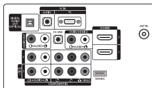
DETAILS DU PANNEAU DES PRISES 7,2"W X 3,7"H
