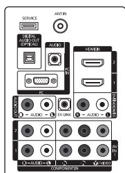
DETAILS DU PANNEAU DES PRISES 4,1"W X 6,4"H
