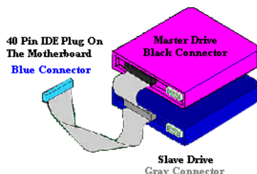
Figure 2-10. Comment connectez la nappe Ultra ATA/66 sur votre carte mère
