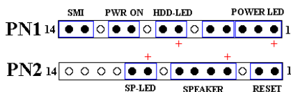
Figure 2-9. définitions des pins du PN1 et PN2
