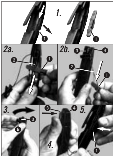
Abb. 6: Mikrofon montieren
