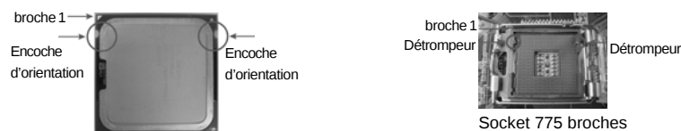
Processeur 775 broches
