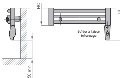
VERSION ELECTRIQUE à liaison infrarouge
